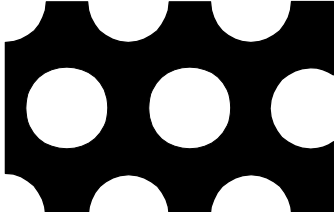
10φ 15P 40.0%
