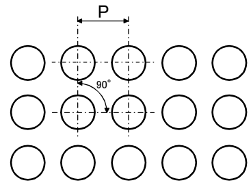
丸穴 平行型
